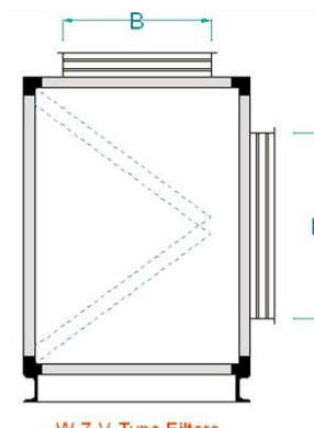
W-Z-V Type Filters
